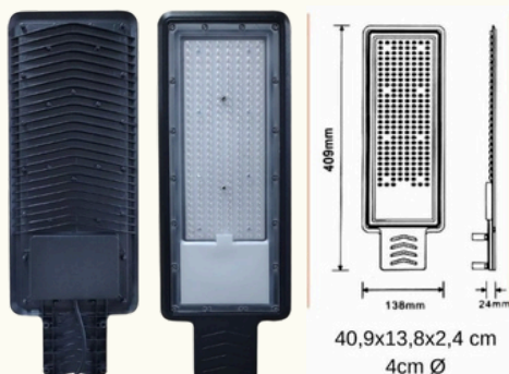
LÚMINARIA PÚBLICA SMD RETANGULAR SLIM IP66 110LM/W 100W BIVOLT PRETO 6500K
